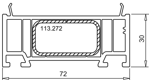
Розширювач - арт. № 114038
