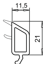
Штапик - арт. № 107218 для склопакета 40мм
