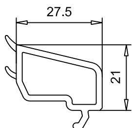
Штапик - арт. № 107143 для склопакета 24мм
