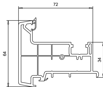
Штульп - арт. № 102340
