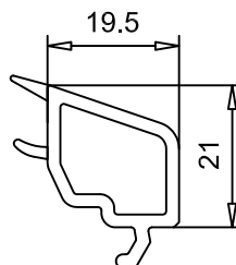
Штапик - арт. № 107215 для склопакета 32мм
