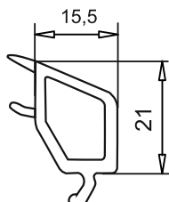
Штапик - арт. № 107217 для склопакета 36мм
