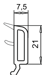
Штапик - арт. № 107228 для склопакета 44мм
