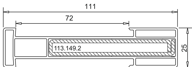
З'єднувач 25 мм арт. № 116228.2
