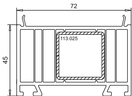
Розширювач - арт. № 114060
